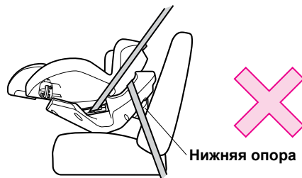
Нижняя опора
