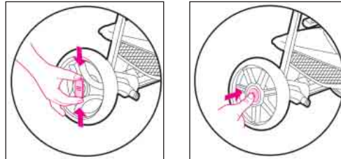
Поворотное колесо свободно
